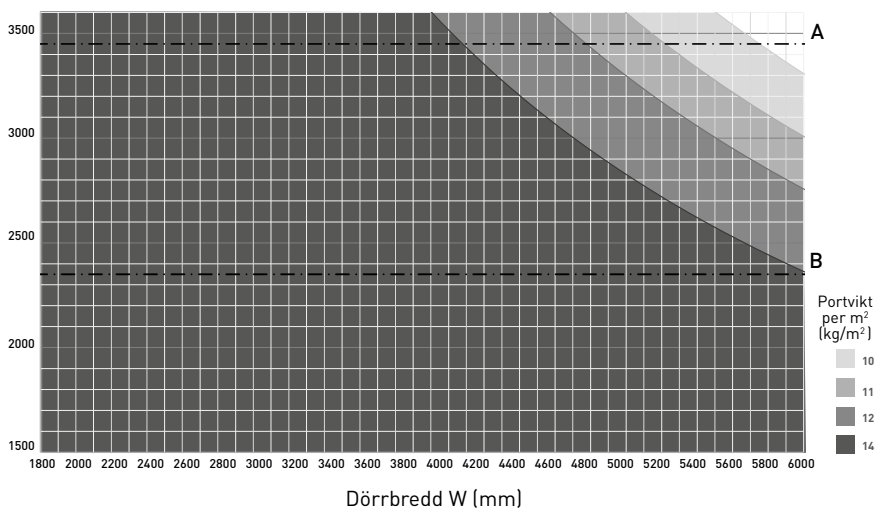
Maximala portmått - SPARK 1000 (maximal portvikt = 200 kg)
