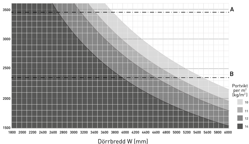
Maximala portmått - SPARK 600 (maximal portvikt = 130 kg)
